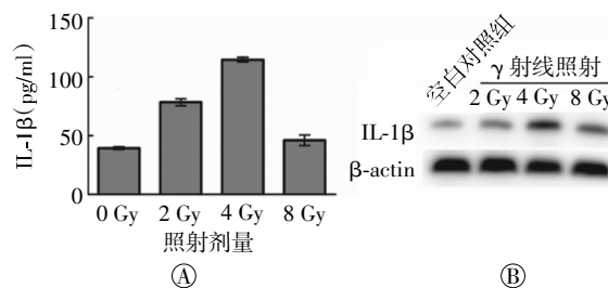
图 1 不同剂量照射后 MSCs IL-1 \beta 的分泌和表达水平 图中，A：给予 MSCs 不同剂量(0、2、4 和 8 Gy)照射，照射后 24 h MSCs 胞外分泌 IL-1 \beta 的变化情况(与空白对照组比较，2 Gy: t = 14.47, P < 0.01 ; 4 Gy: t = 16.33, P < 0.01 )；B：MSCs 受照后 24 h 胞内 IL-1 \beta 蛋白的表达改变。MSCs：间充质干细胞。
