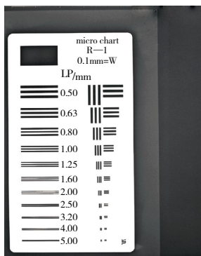
图 1 应用自动曝光控制模式的 X 线用矩形波测试卡测试结果 摄影条件为 158 mAs 时，辐射剂量达到 3.0 mGy，X 线用矩形波测试卡可观察到 4 LP/mm。
