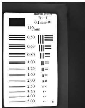
图 2 应用手动曝光控制模式的 X 线用矩形波测试卡测试结果 摄影条件为 80 mAs 时，辐射剂量只有 1.5 mGy，X 线用矩形波测试卡仍可观察到 4 LP/mm。
